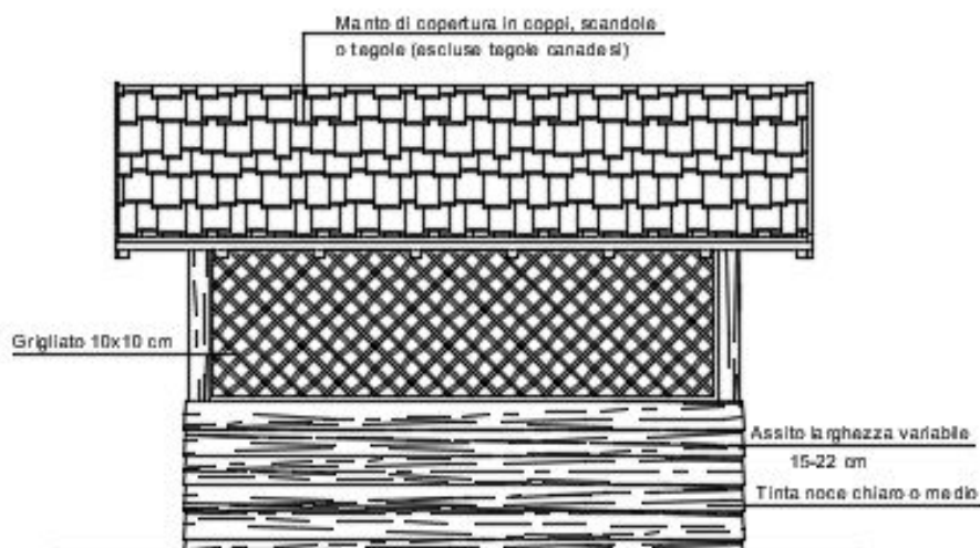
VISTA LATERALE
