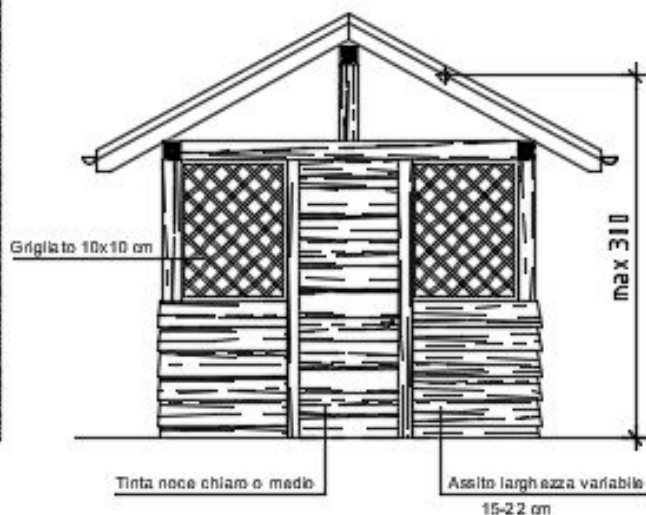
VISTA FRONTALE
