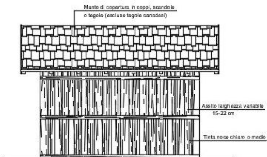
VISTA LATERALE
